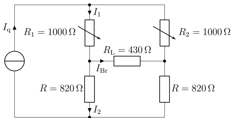
Abbildung 2.5: Beispiel für ein mittels CircuiTikZ erstelltes Schaltbild (siehe auch https://www.overleaf.com/read/pnmjpycmmhgx )
