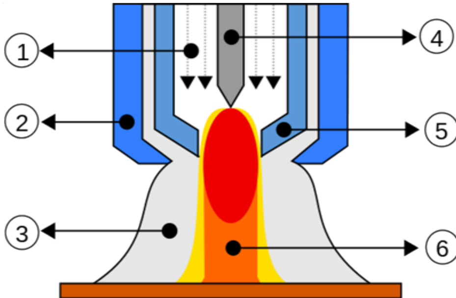
Şekil 4.2 PTA Torç
