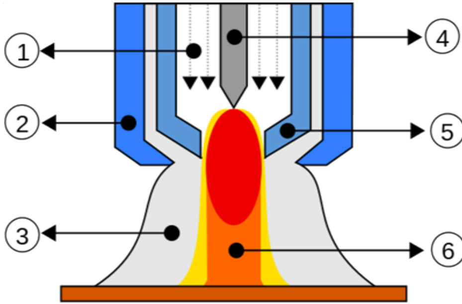
Şekil 1.1 PTA Torç
