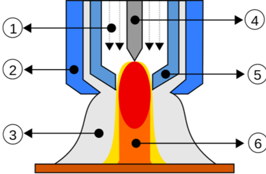
Şekil 2.4 PTA Torç
