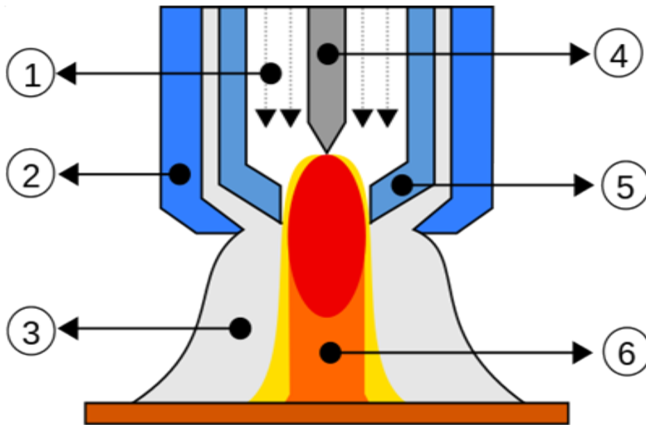
Şekil 4.3 PTA Torç
