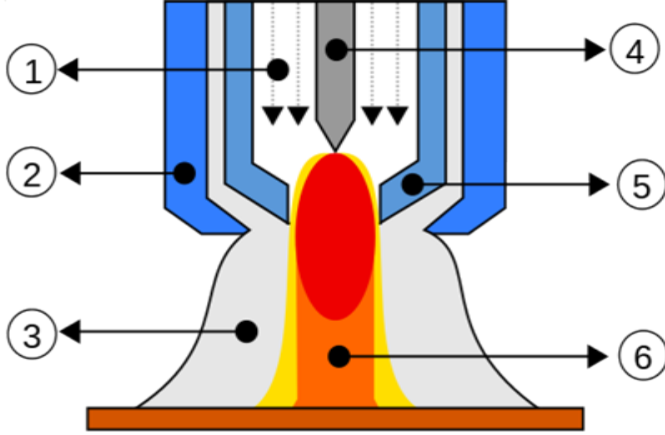
Şekil 5.1 PTA Torç
