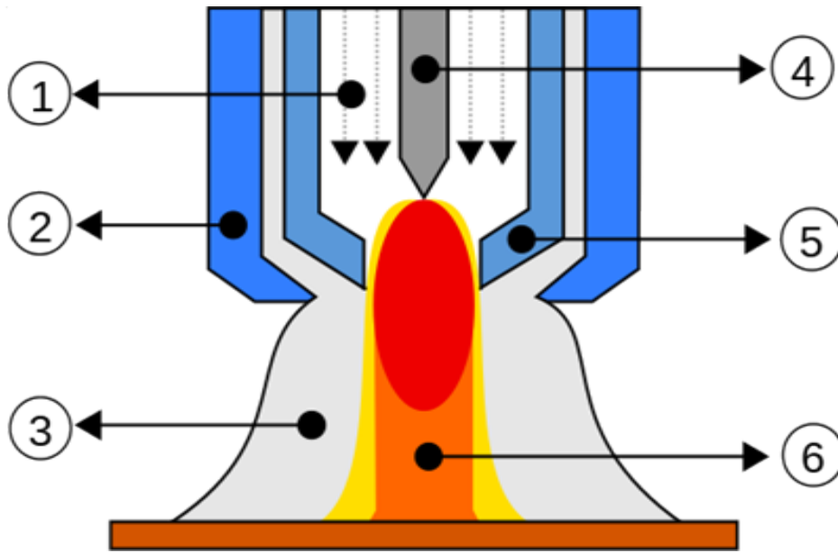
Şekil 1.3 PTA Torç
