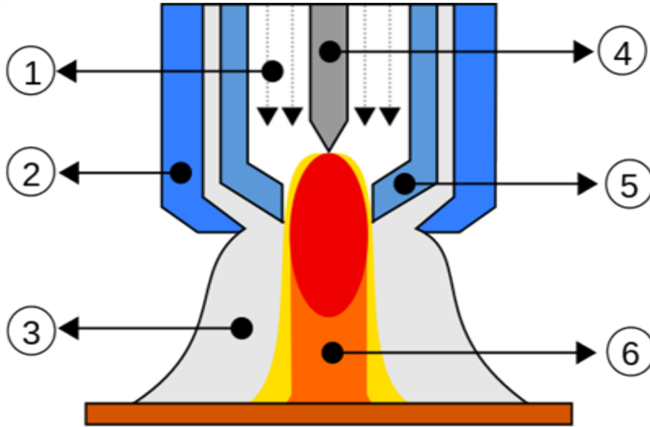
Şekil 2.3 PTA Torç
