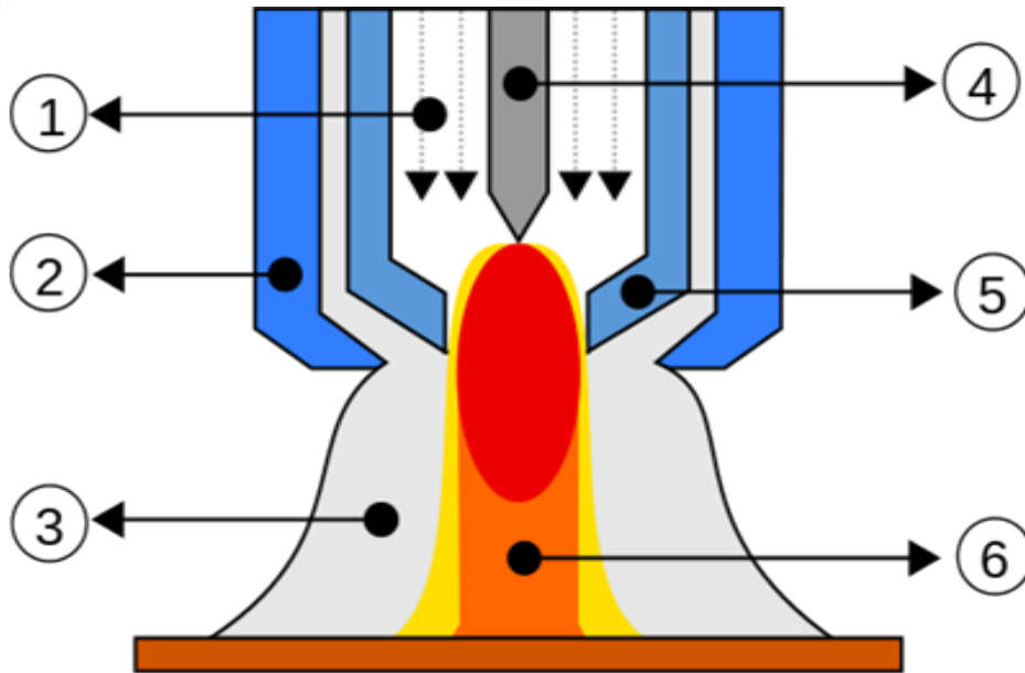
Şekil 3.3 PTA Torç
