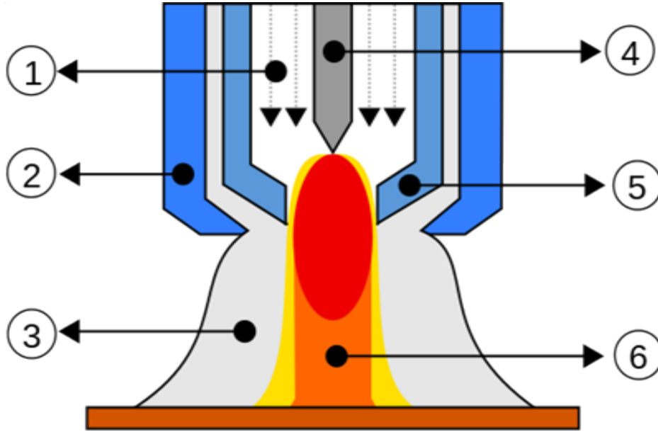
Şekil 5.4 PTA Torç
