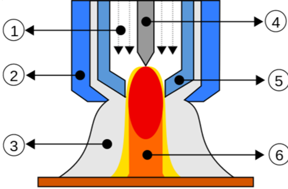
Şekil 3.1 PTA Torç
