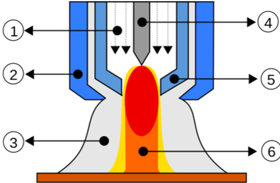
Şekil 5.2 PTA Torç
