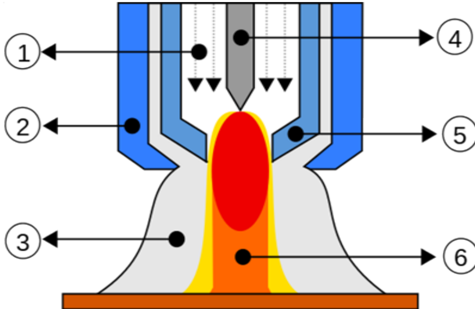
Şekil 1.2 PTA Torç
